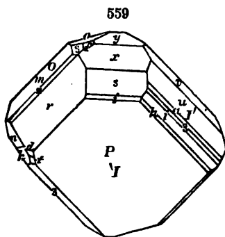
Dauphiny.
